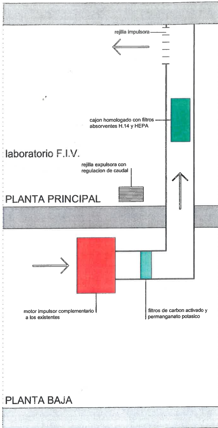
ESQUEMA DE LA LINEA DE AIRE AMBIENTAL A PRESION POSITIVA, ULTRALIMPIO, PARA LABORATORIO DE F.I.V. (ZONA ULTRALIMPIA ESPECIAL) COMPLEMENTARIA A LA EXISTENTE
